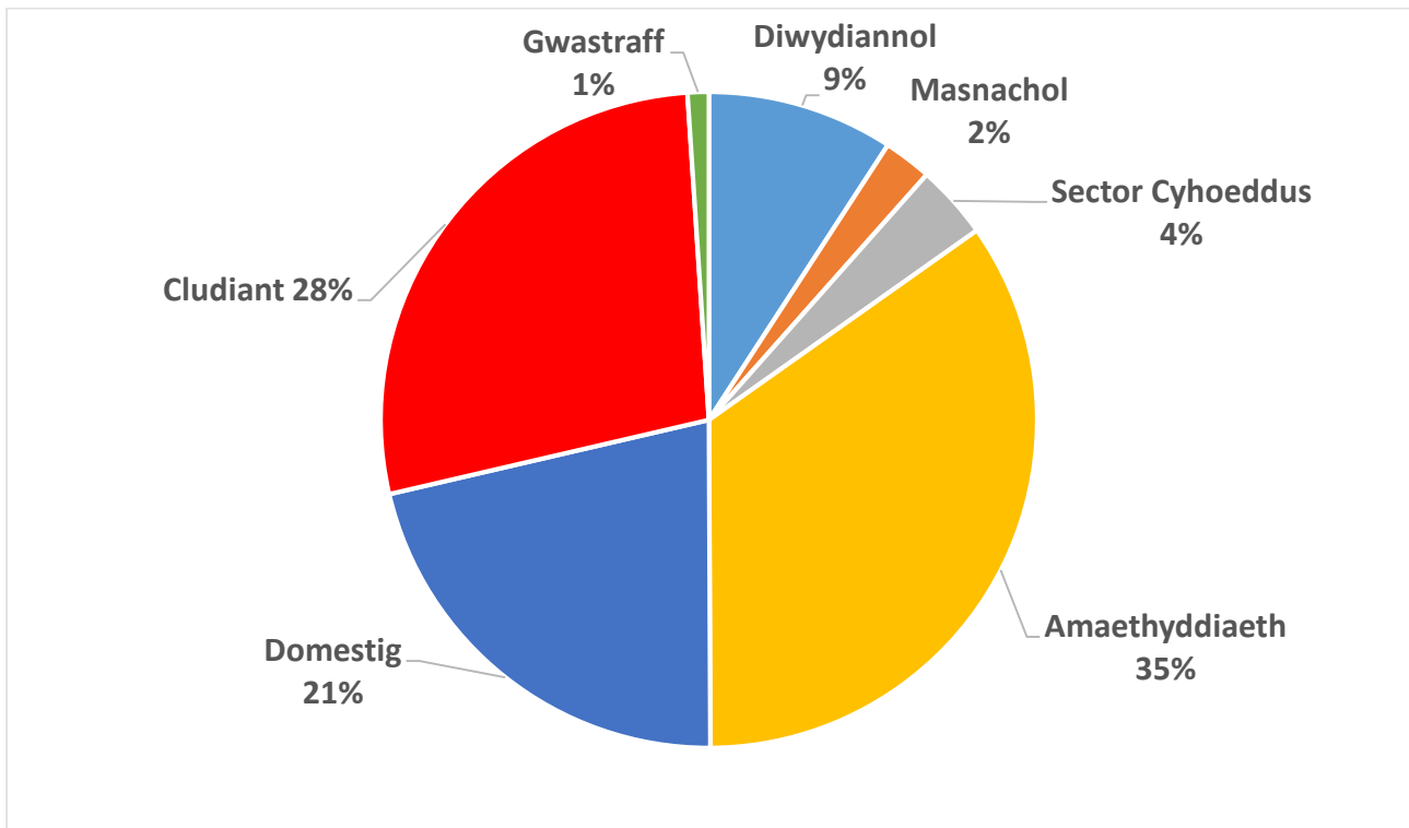
Siart 11: Ôl-troed Carbon Sir Ddinbych yn 2021/22 (kt CO 2 e)
