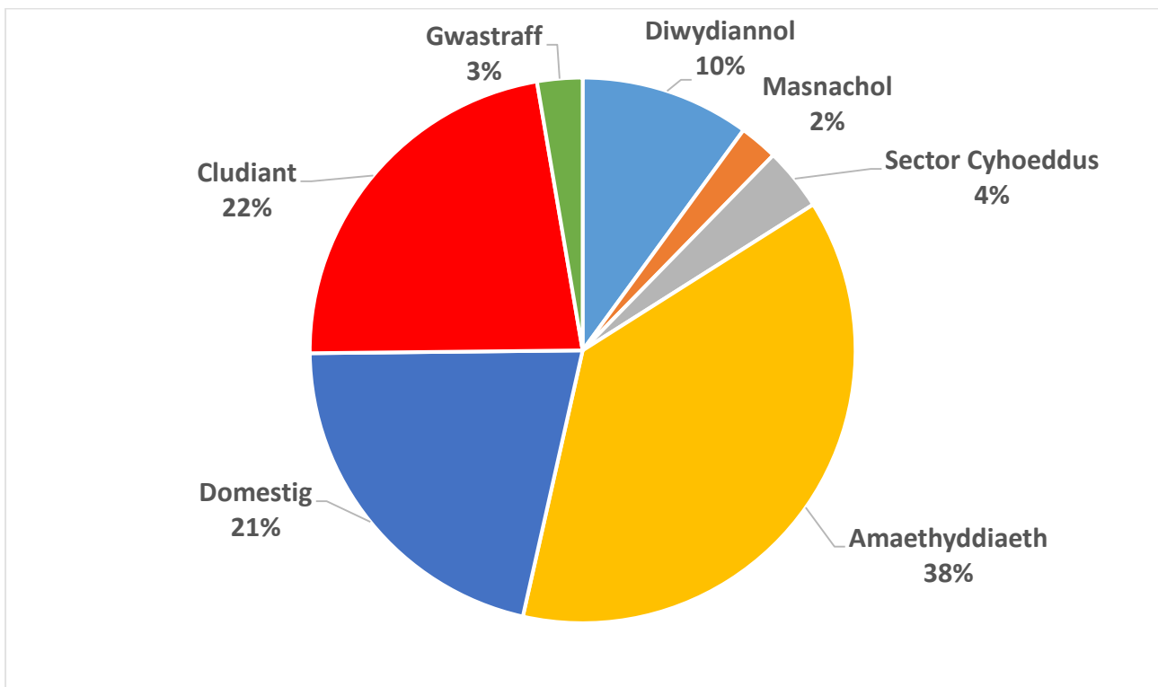
Siart 11: Ôl-troed Carbon Sir Ddinbych yn 2021/22 (kt CO 2 e)
