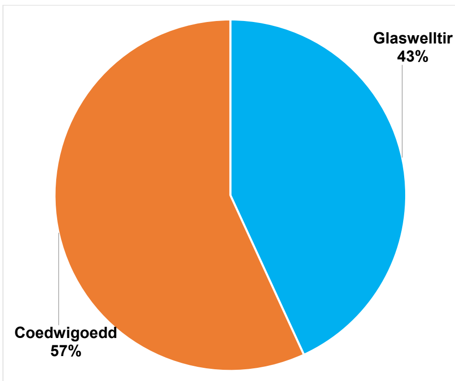
Siart 4: Amsugnad Carbon Cyngor Sir Ddinbych yn 2022/23
